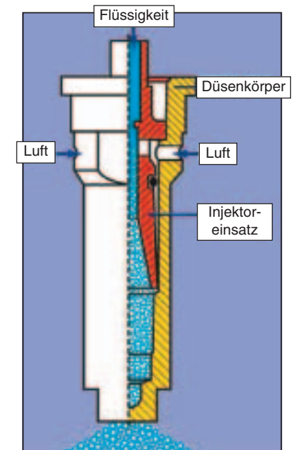
Innovative Lösung: Injektordüsen für Feldspritzgeräte minimieren die Abdrift bis zu 90 Prozent.
