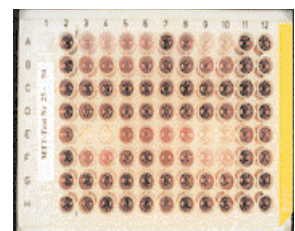
MTT-Zellkultur-Test
